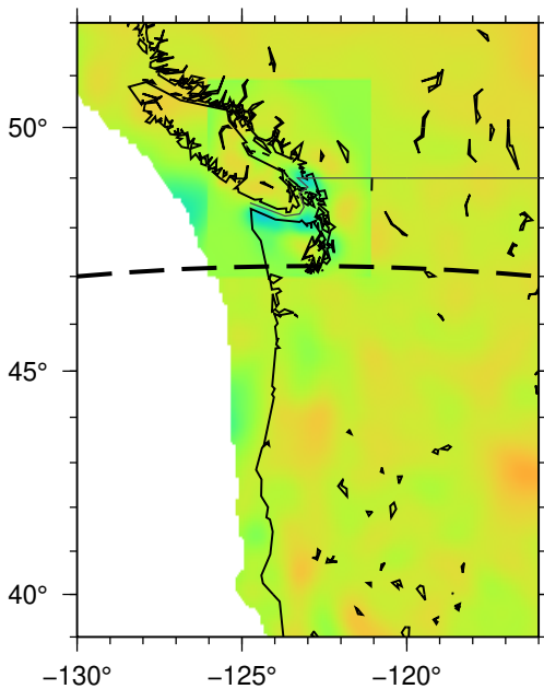
(d) Vp aggregate: z = 2 km
