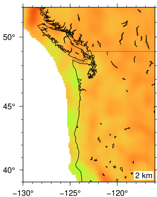
(d) WUS324 Cascadia: Original
