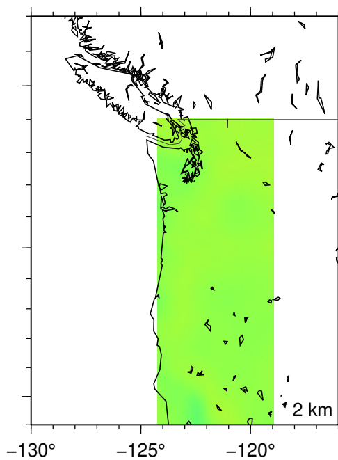
(d) WUS324 Cascadia: Original
