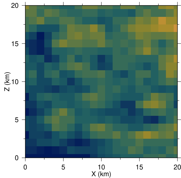
(d) Vs Perturbed: y = 10 km
