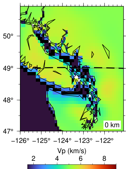
(d) Original Vp
