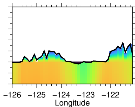
(h) Linear Vs
