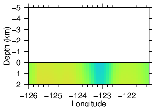
(g) Linear Vp
