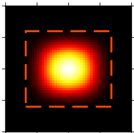
(44) Agnesi
