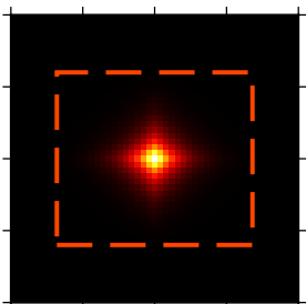
(31) Riemann
