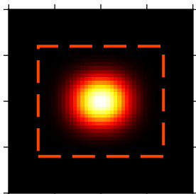
(33) Connes
