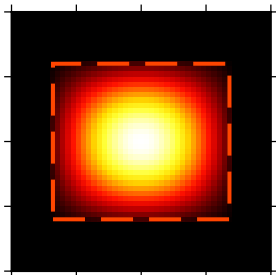
(39) Tanh
