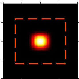
(34) Kaiser-Bessel
