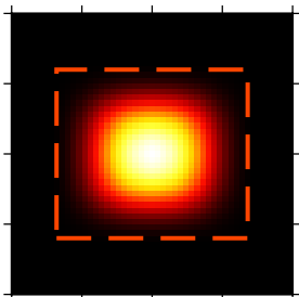
(45) Inverse quadratic
