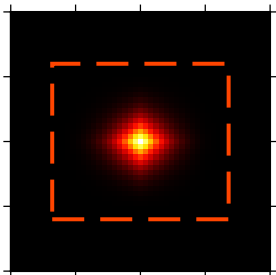
(40) Erf
