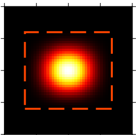
(32) Fejer
