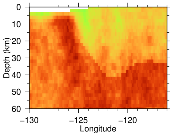
(d) WUS324 Cascadia: Perturbed
