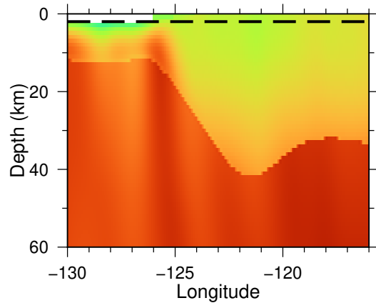
(d) Vp aggregate: latitude = 47 N
