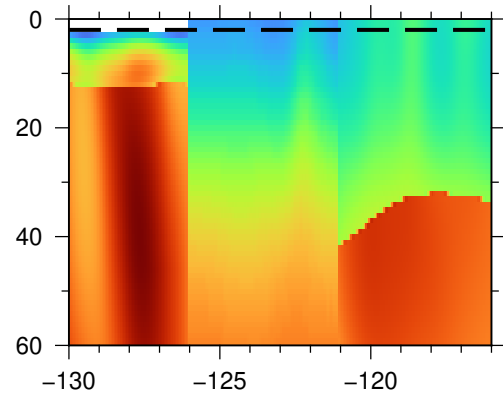
(c) Density tiling: latitude = 47 N
