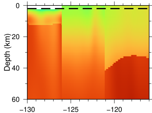
(a) Vp tiling: latitude = 47 N
