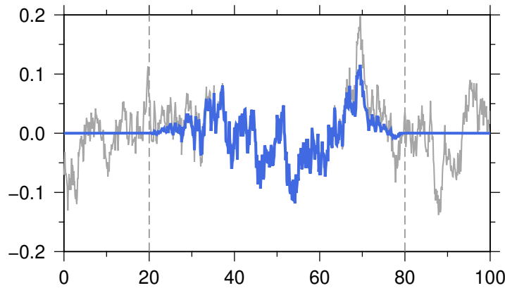
(d) Smoothstep
