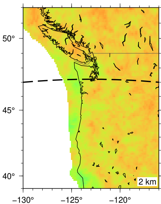
(d) WUS324 Cascadia: Perturbed
