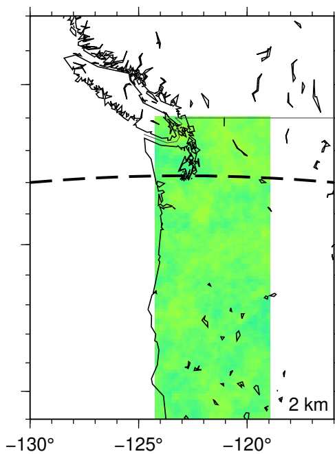
(d) WUS324 Cascadia: Perturbed
