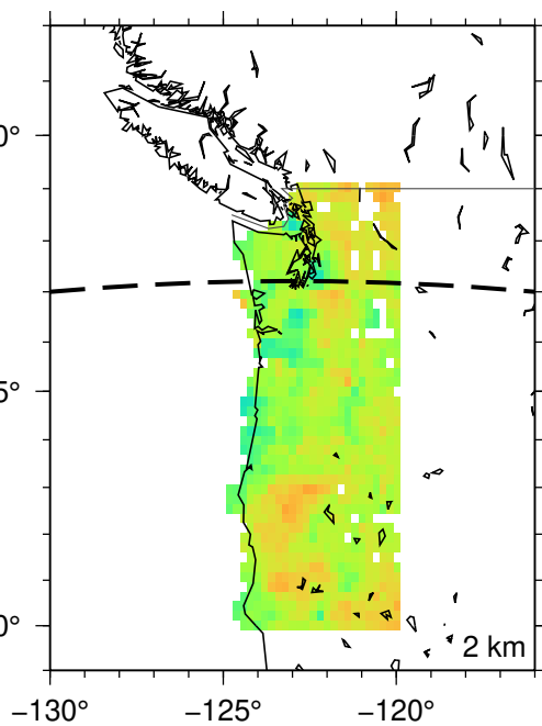
(d) WUS324 Cascadia: Perturbed
