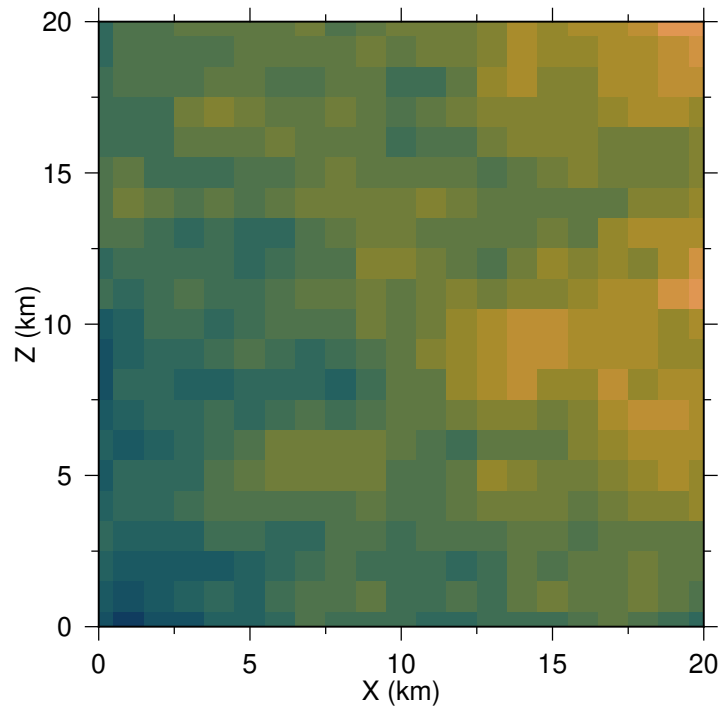
(d) Vp Perturbed: y = 10 km
