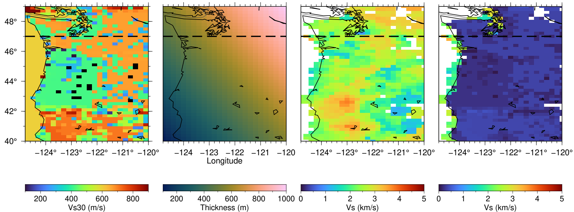
(a) USGS Vs30
