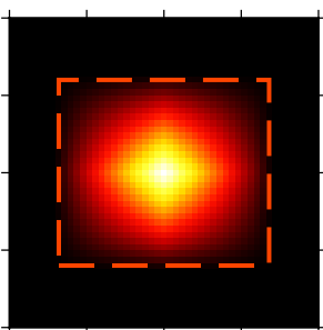
(8) Parzen
