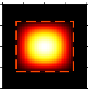
(18) Quadratic
