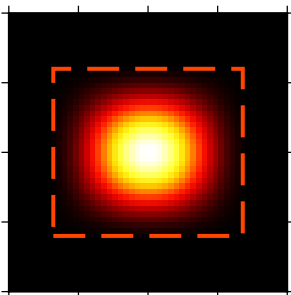
(21) Bartlett-Hann
