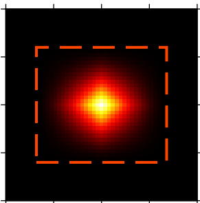
(23) Hanning-Poisson
