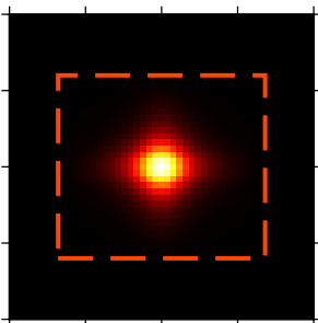
(22) Lanczos
