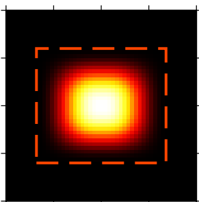
(16) Kaiser
