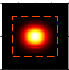
(14) Bohman
