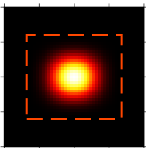
(13) Sine
