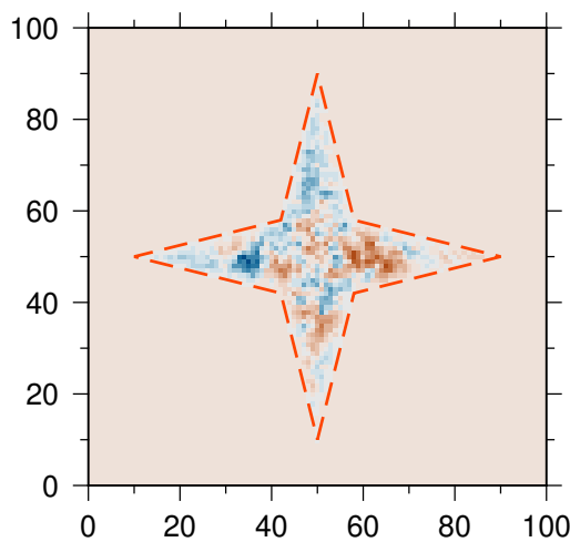
(b) Linear
