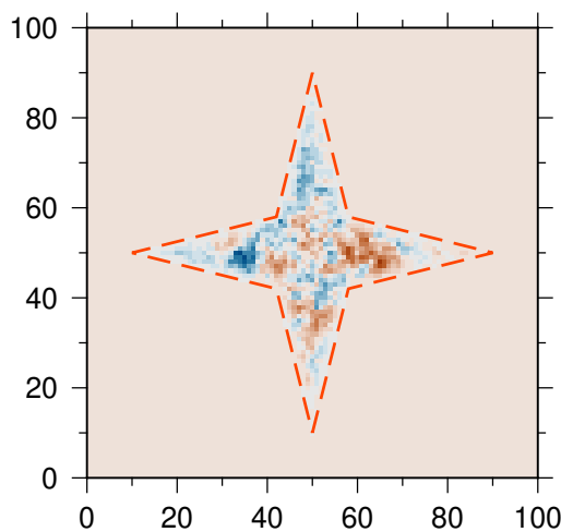
(d) Smoothstep
