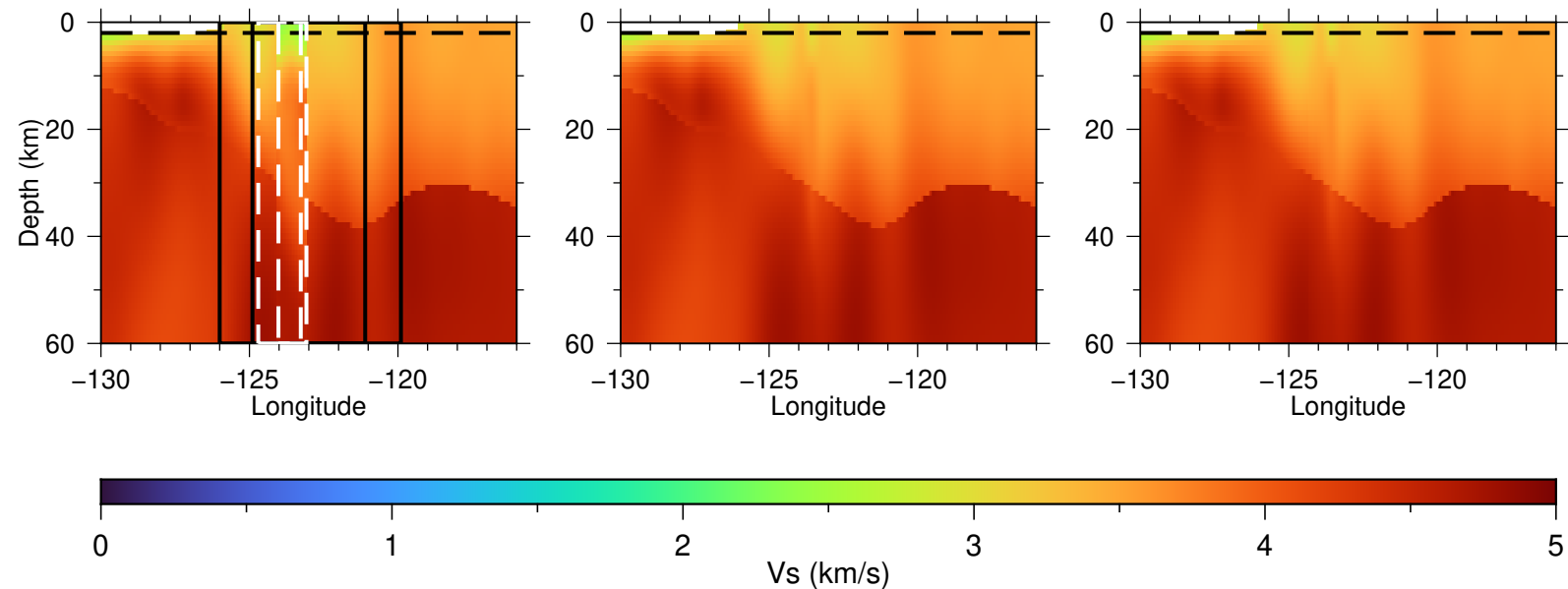
(a) Supported tiling: latitude = 48 N
